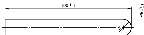
图 11 8 mm 直径的测试指
